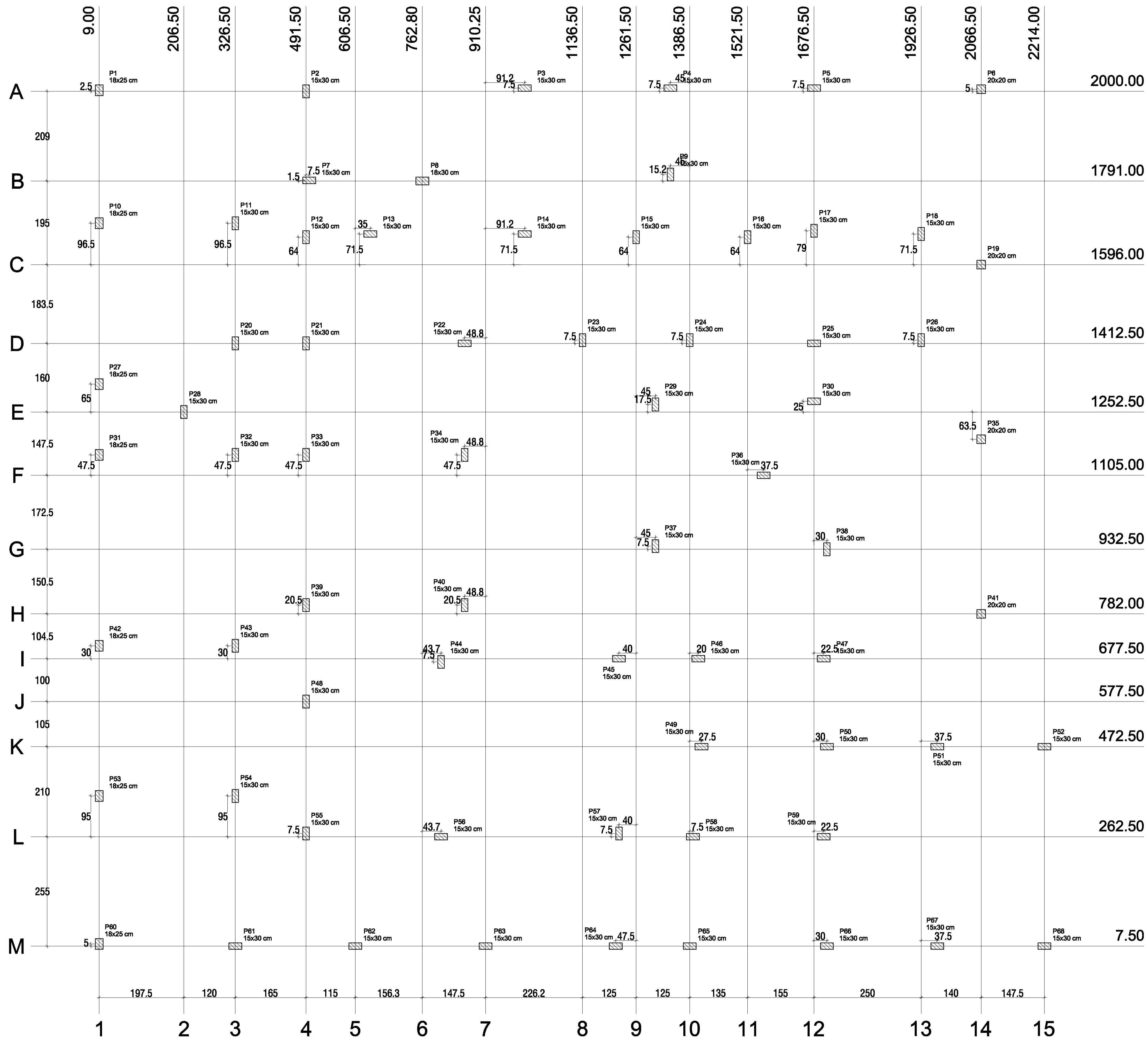
Planta de cargas escala 1:50
