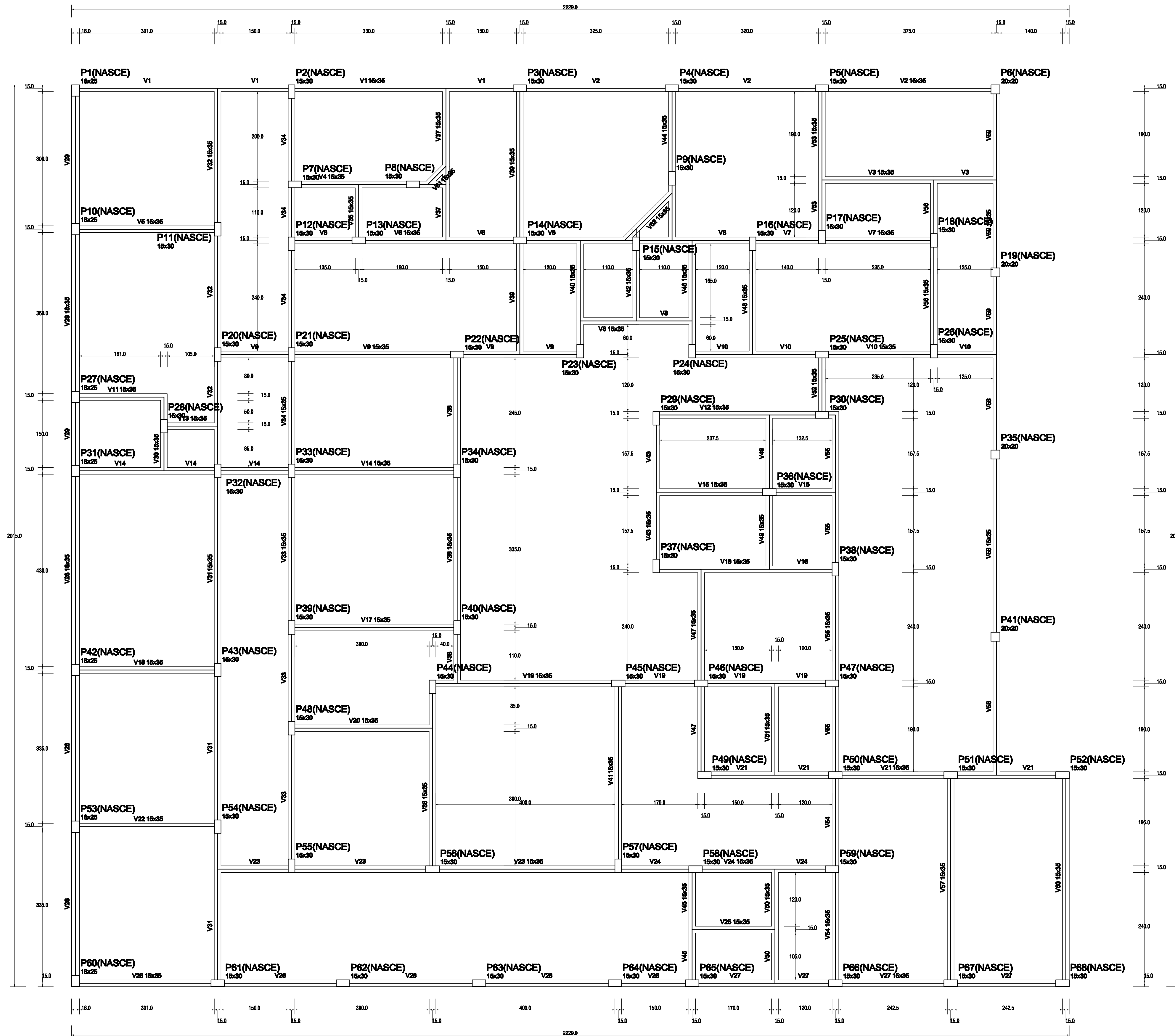
Forma do pavimento Baldrame escala 1:50
