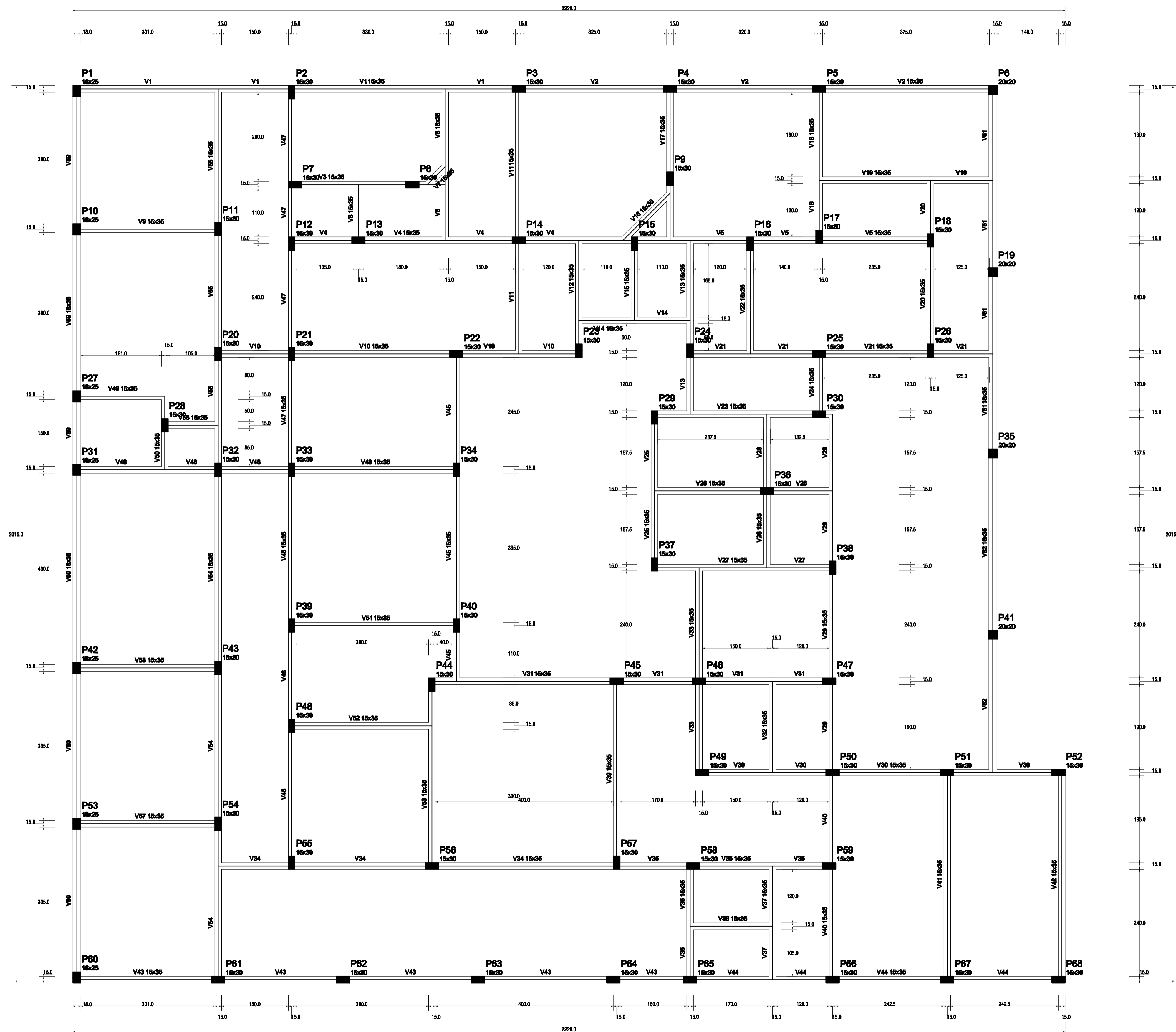
Forma do pavimento Cobertura escala 1:50
