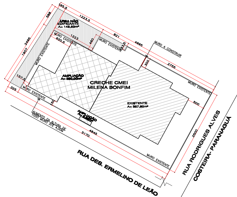
PLANTA DE SITUAÇÃO ESCALA - 1:500
