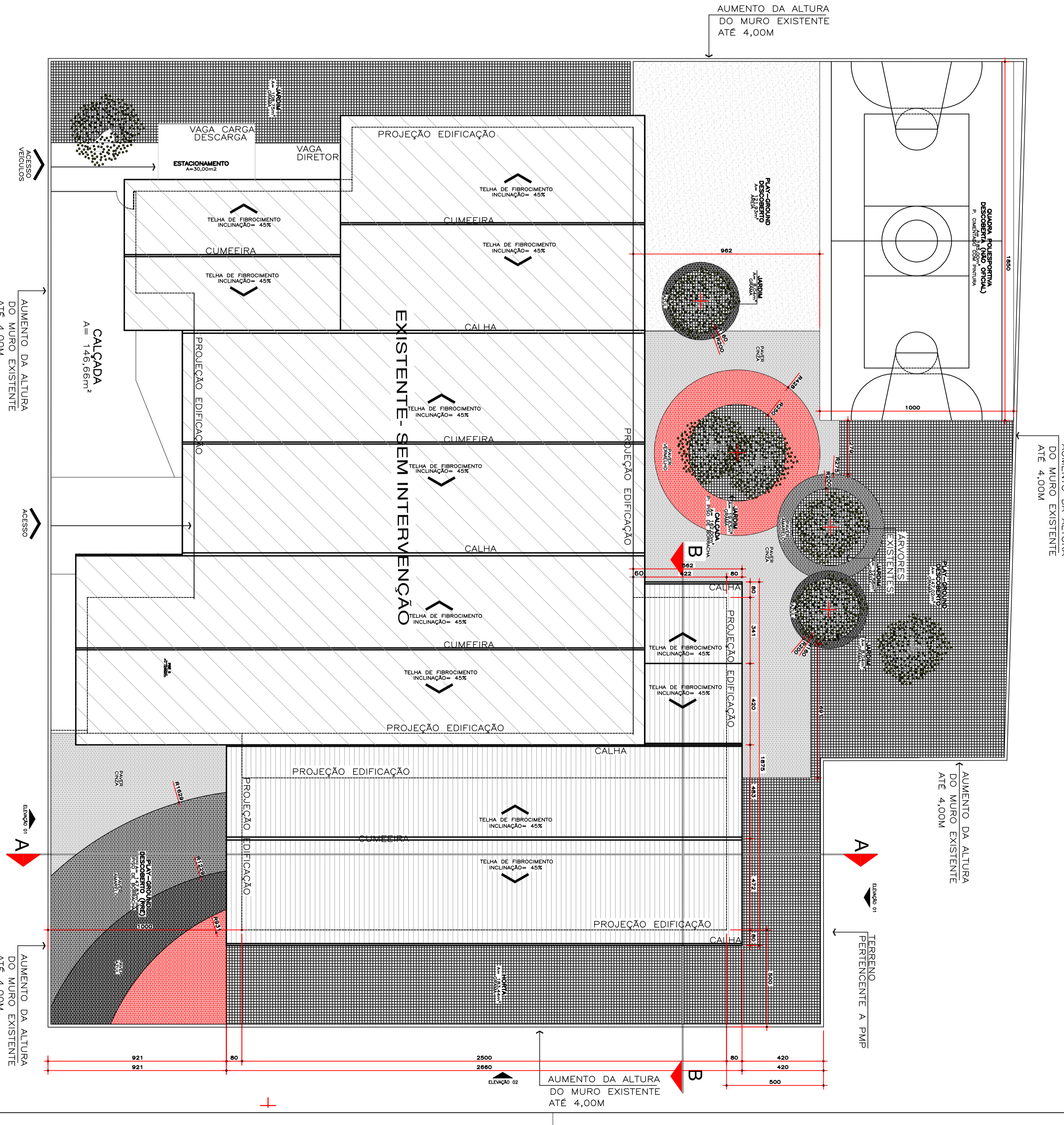
IMPLANTAÇÃO/ PLANTA DE COBERTURA ESCALA - 1/150
