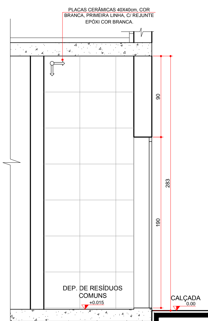
SECCÃO BB ABRIGO DE RESÍDUOS ESCALA 1:25
