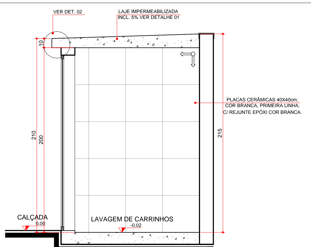
SECCÃO BB LAV. DE CARRINHOS ESCALA 1:25
