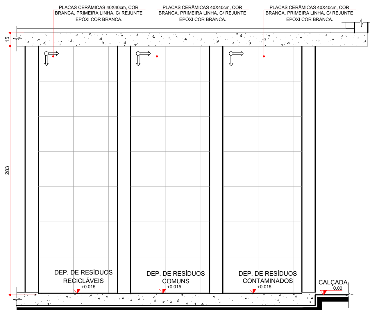
SECCÃO AA ABRIGO DE RESÍDUOS ESCALA 1:25
