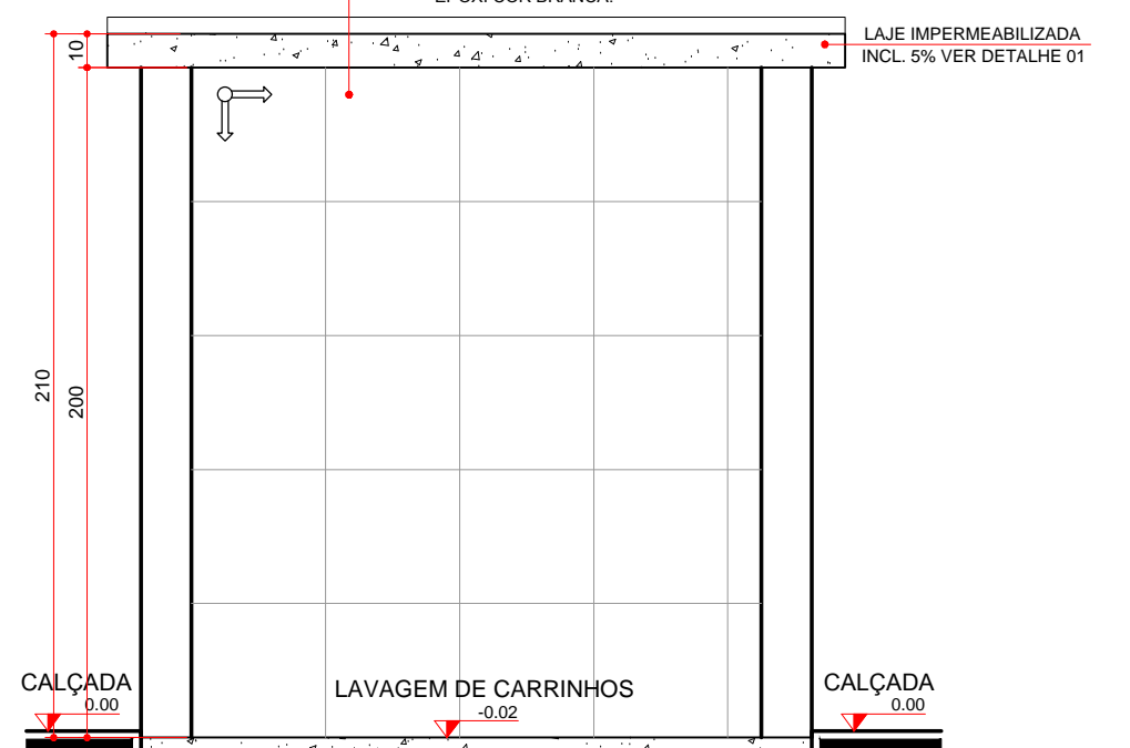
SECCÃO AA LAV. DE CARRINHOS ESCALA 1:25
