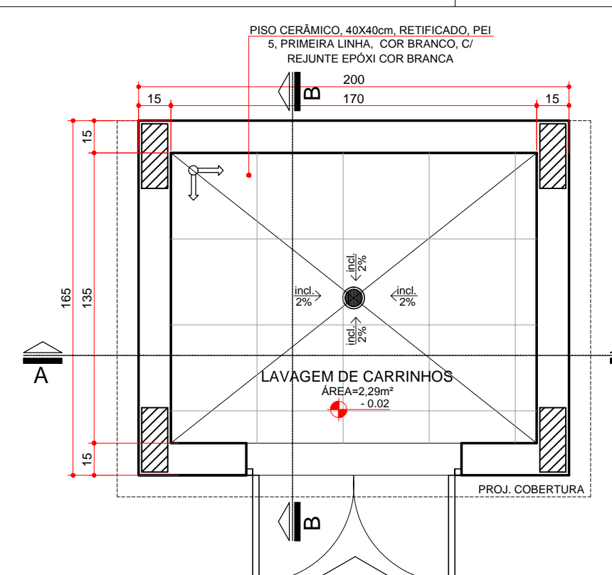
PLANTA BAIXA LAV. DE CARRINHOS ESCALA 1:25
