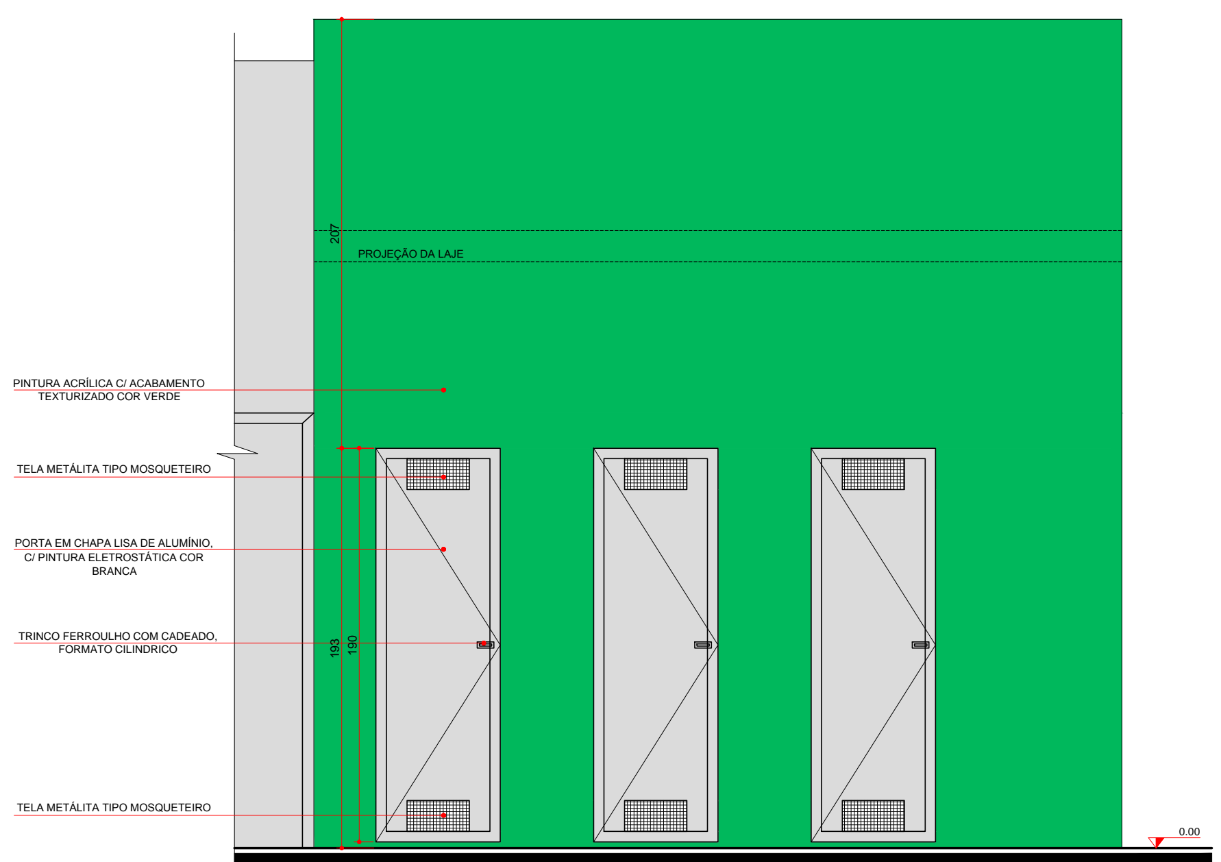
ELEVÇÃO 01 ABRIGO DE RESÍDUOS ESCALA 1:25
