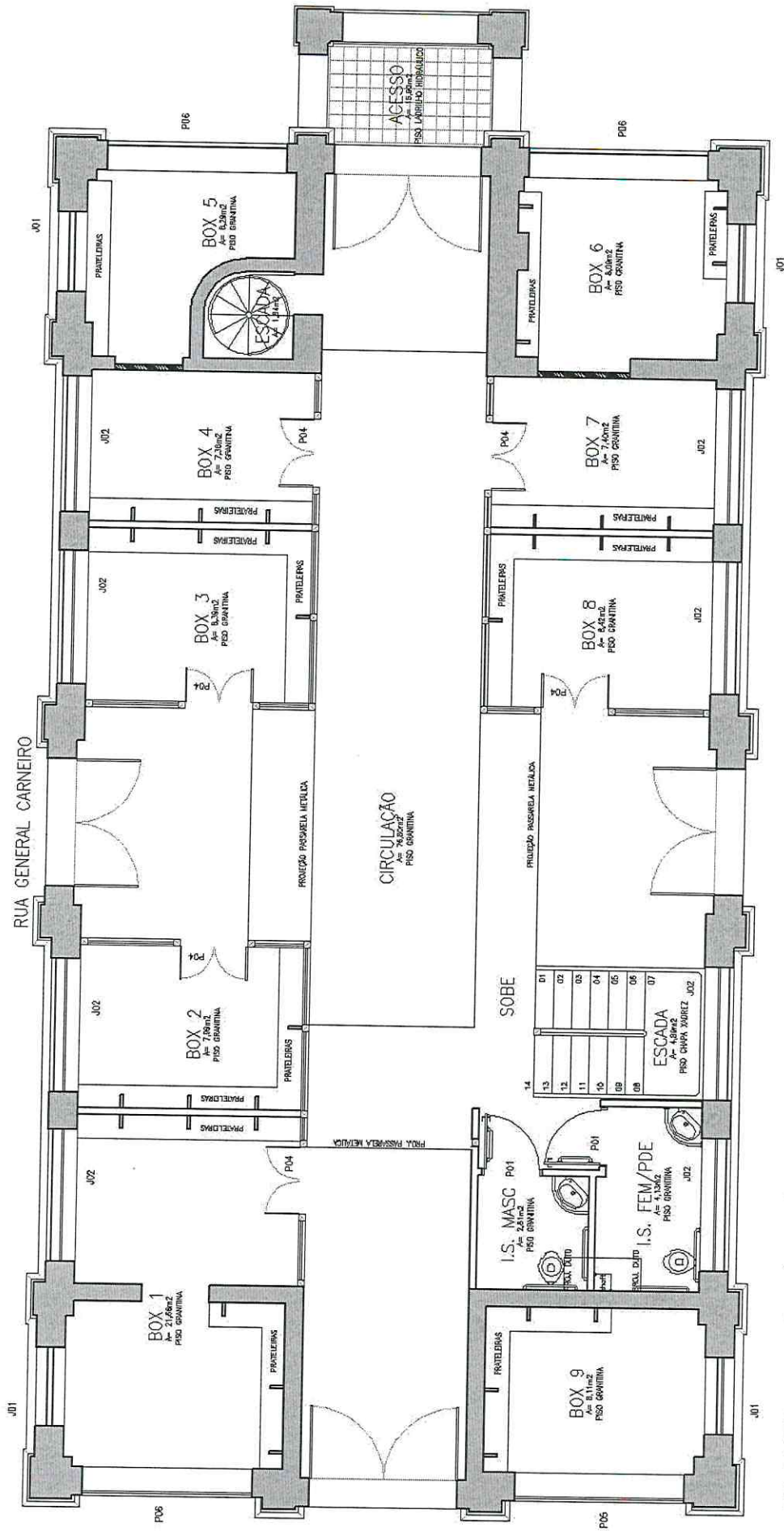
PLANTA PAVTO. TÉRREO
