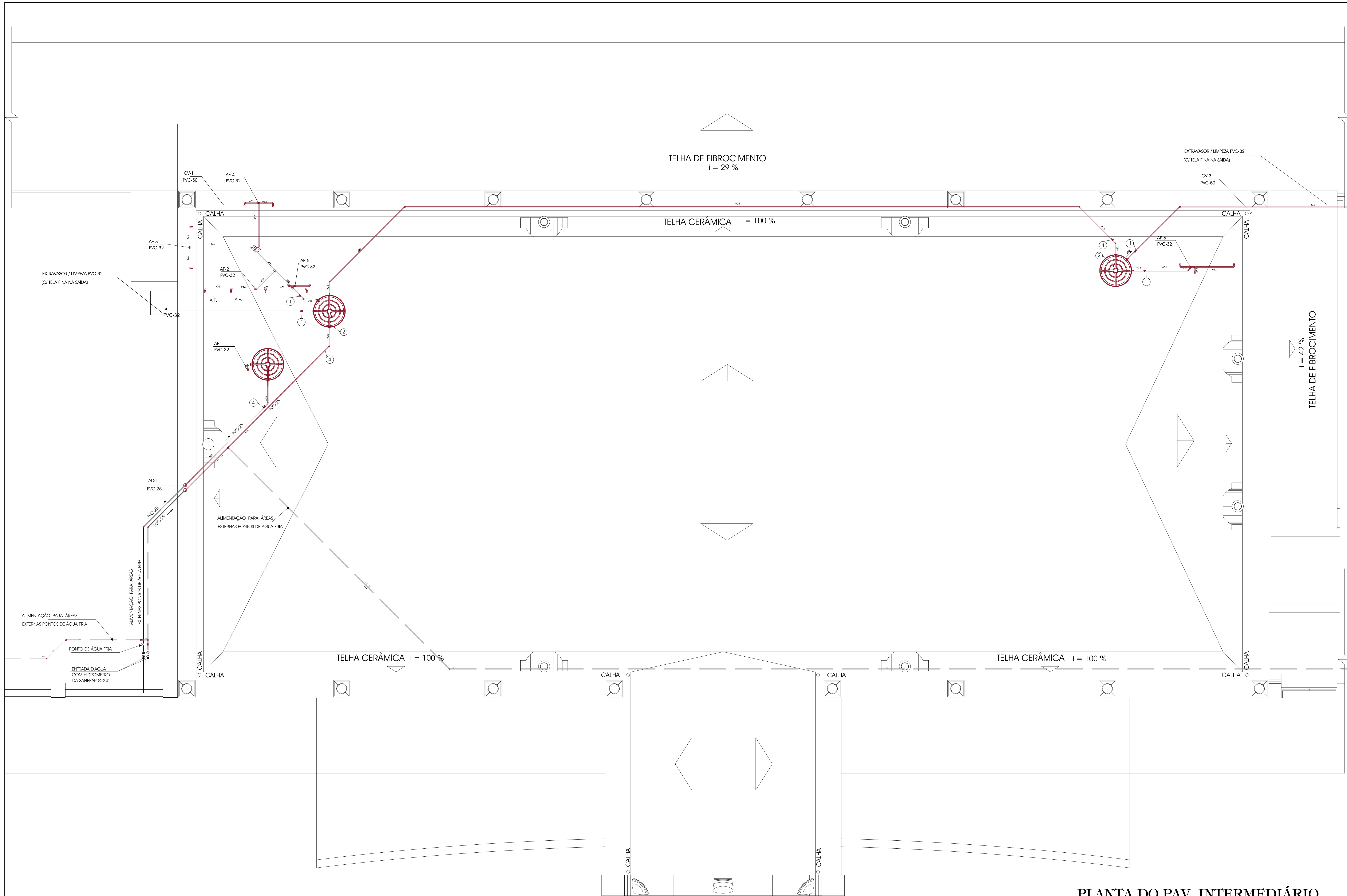
PLANTA DO PAV. INTERMEDIÁRIO ESCALA 1:50
