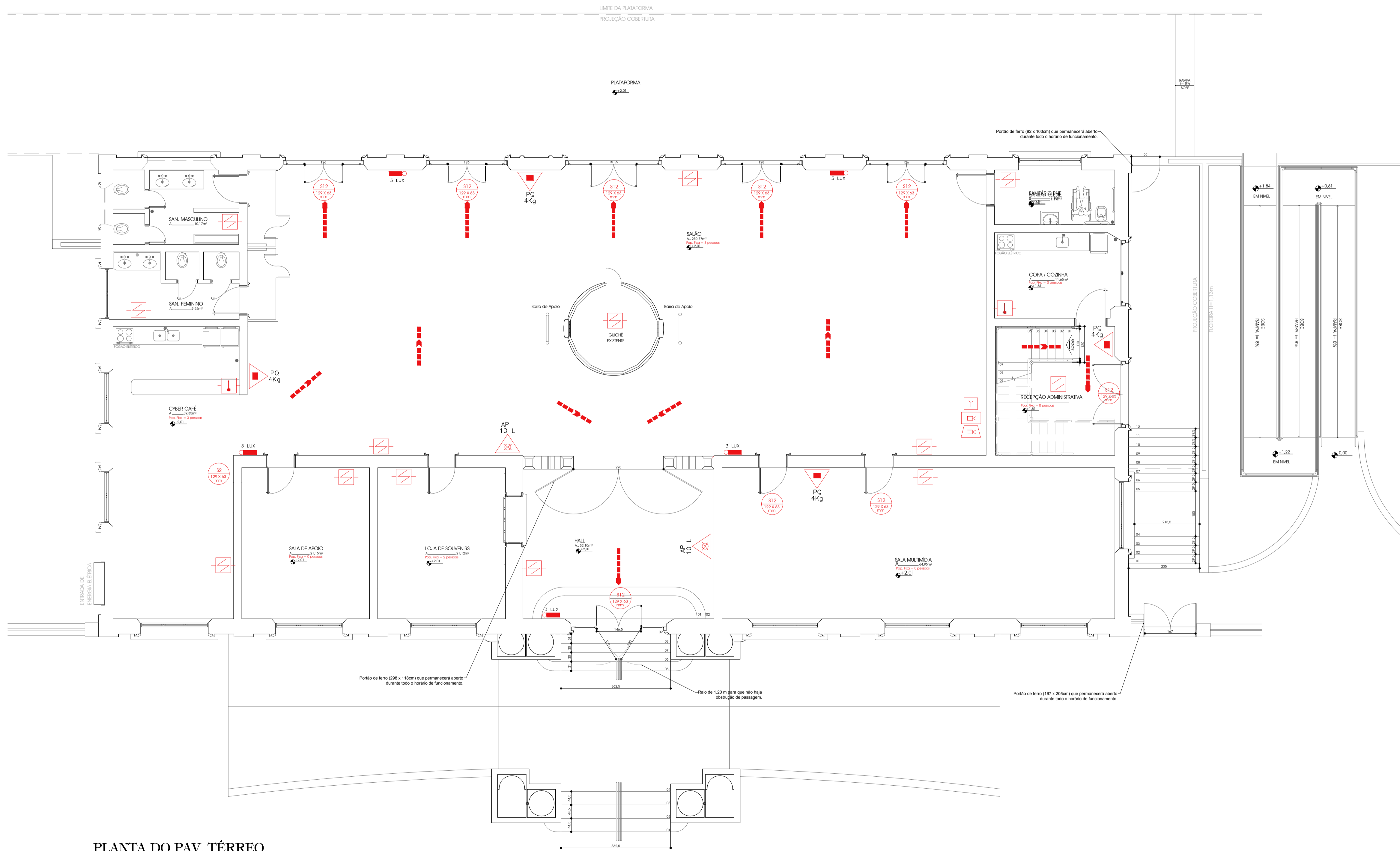
PLANTA DO PAV. TÉRREO ESCALA 1:75
