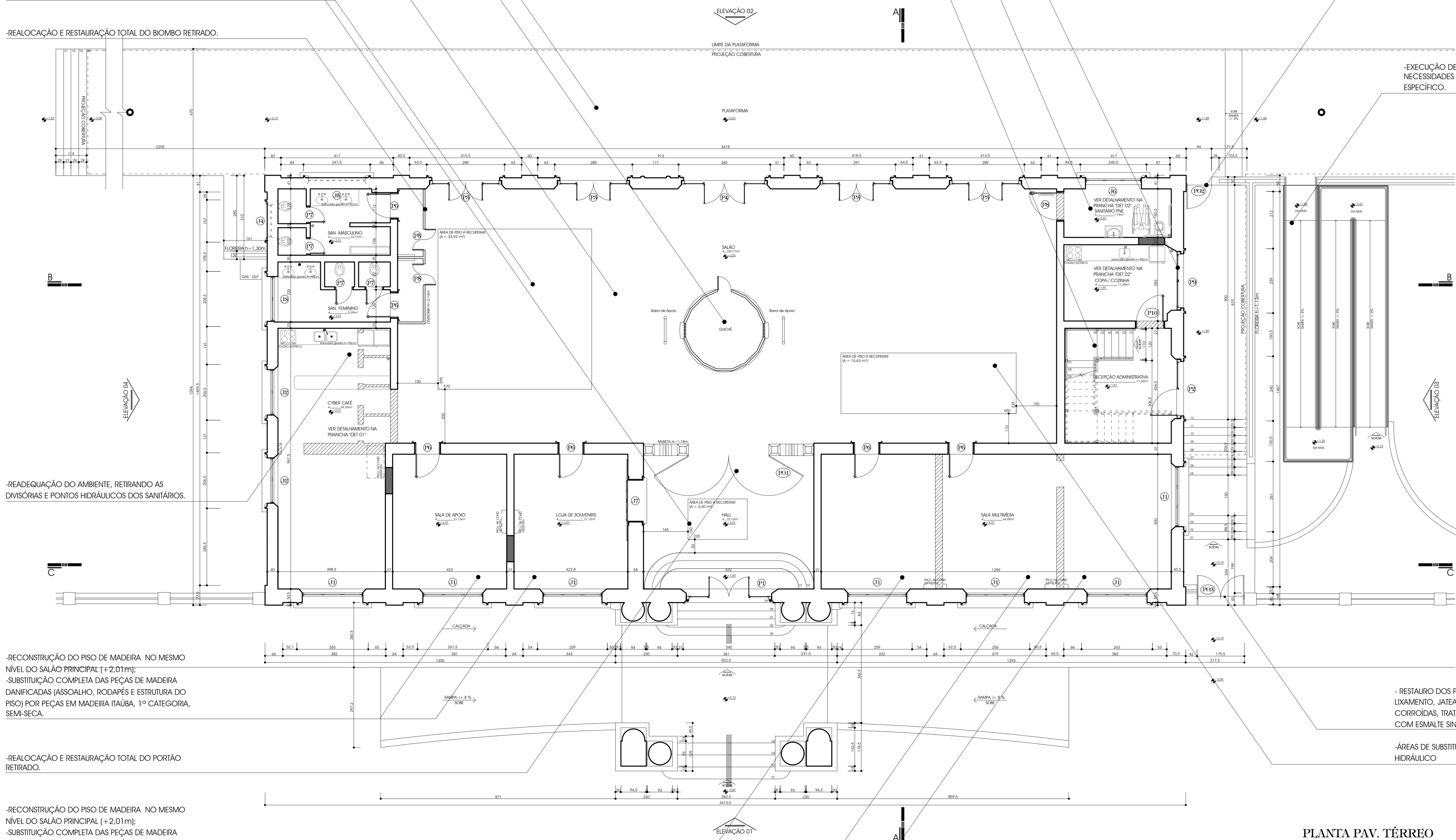
PLANTA PAV. TÉRREO ESCALA 1:75
