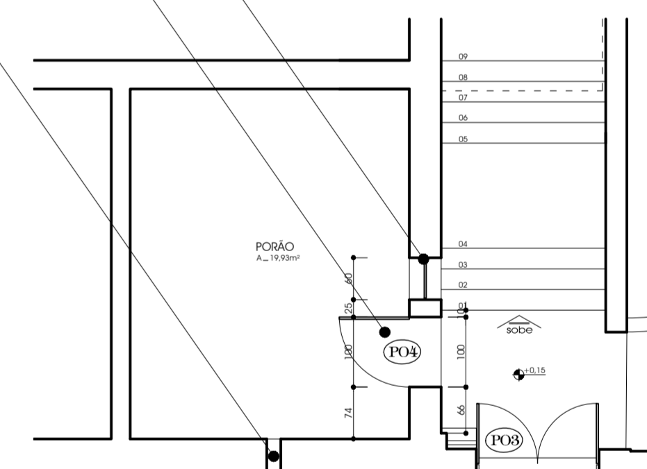
PLANTA PORÃO ESCALA 1:75
