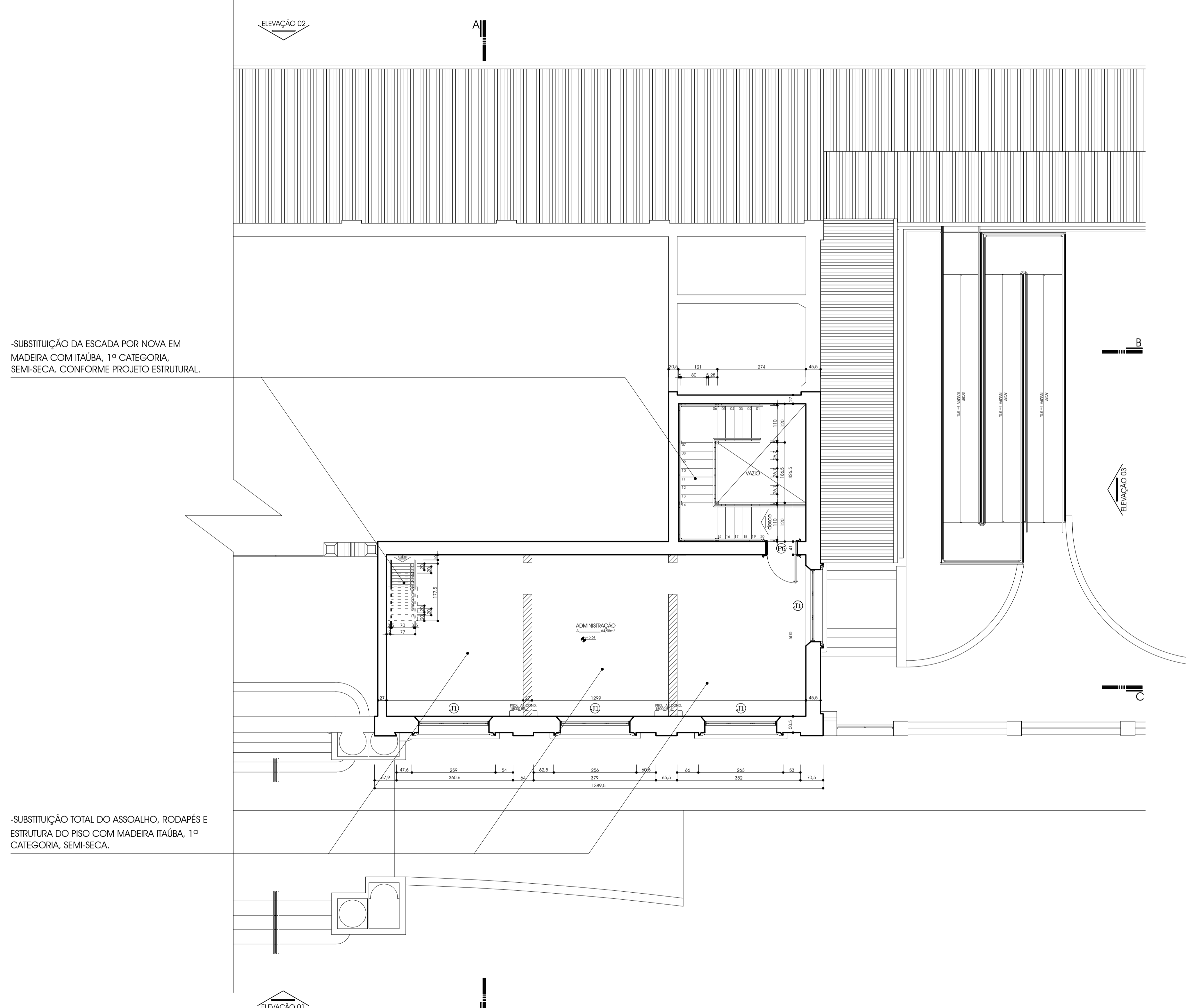
PLANTA PAV. SUPERIOR ESCALA 1:75 PROPRIETÁRIO: _____ PAREDE EXTERNE EM ALVENARIA _____ PAREDE A COBRIR EM ALVENARIA _____ PAREDE A DEMOLIR _____
