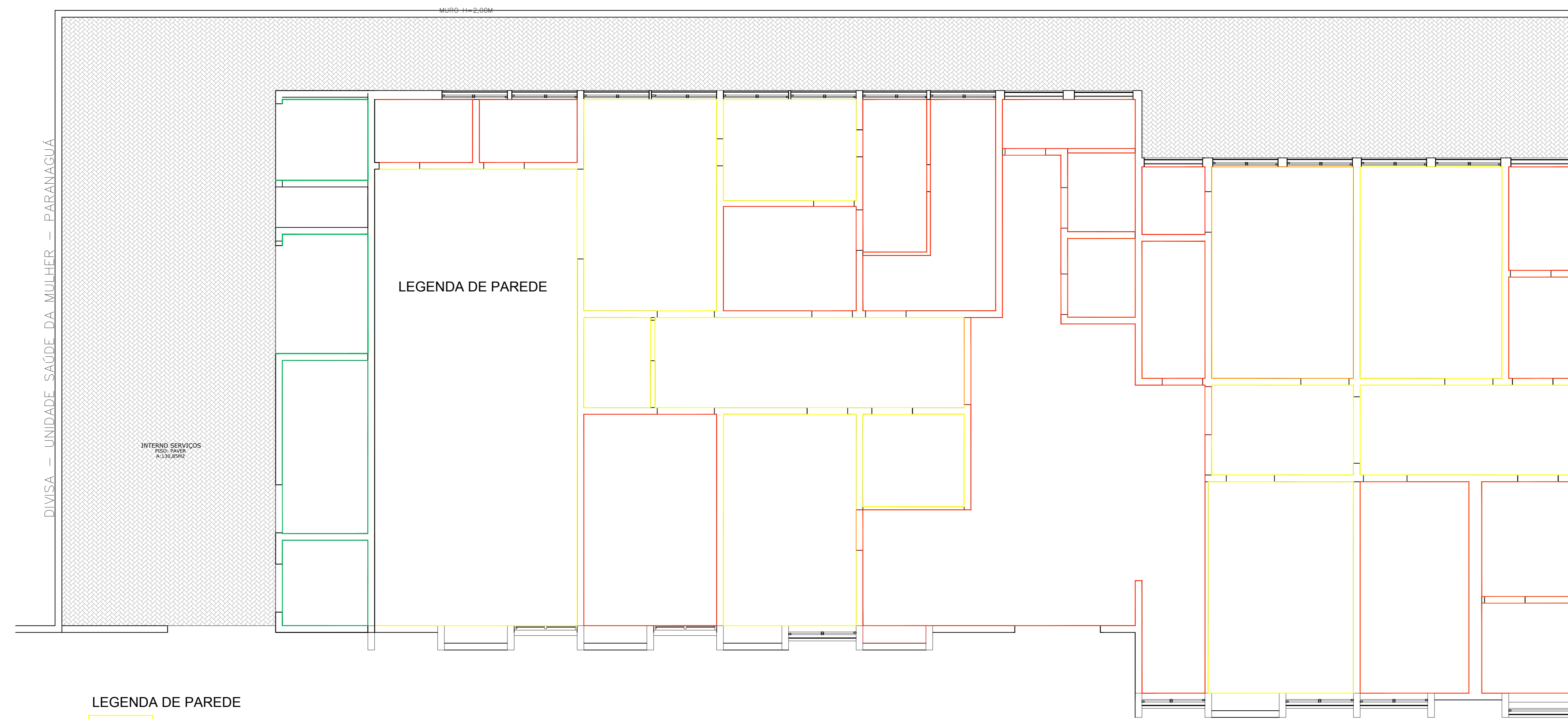
DETALHAMENTO - PINTURA PAREDES Esc.: 1:50
