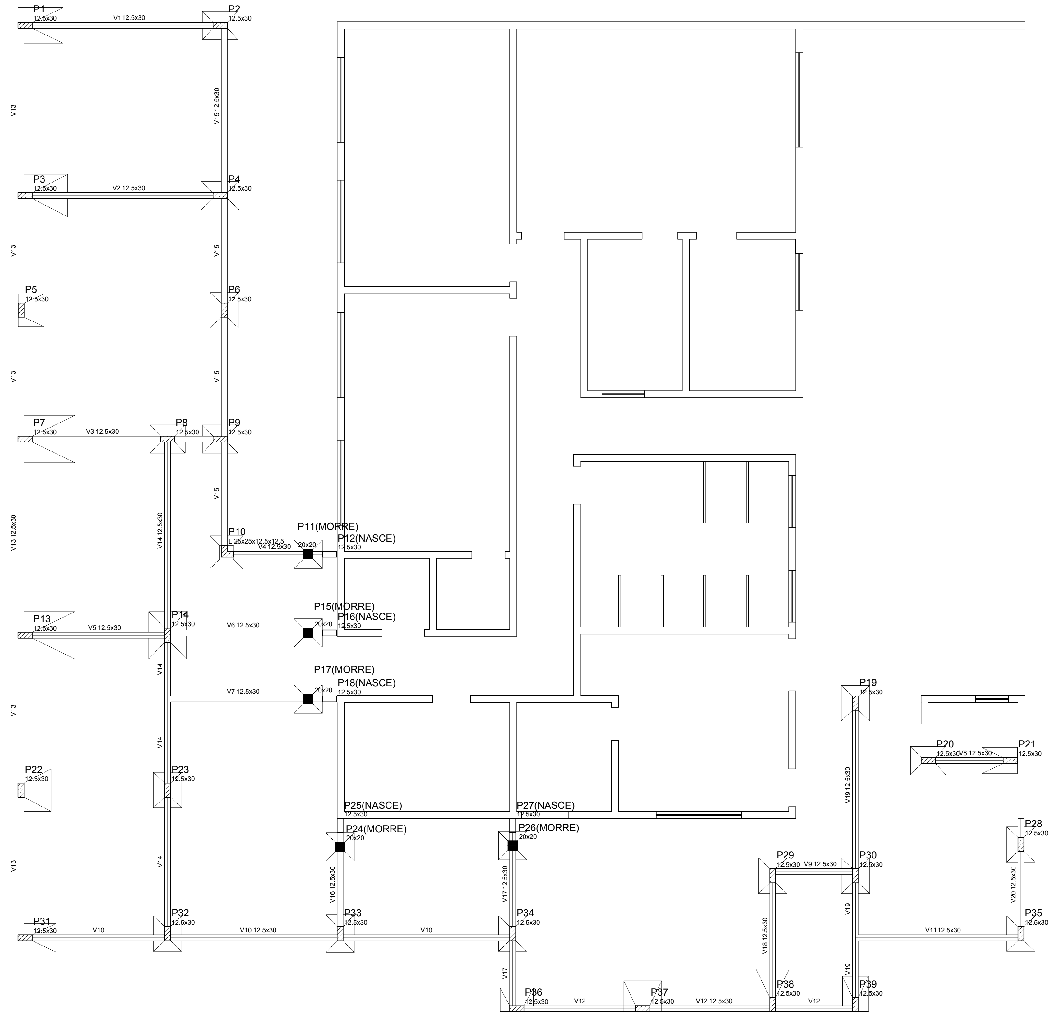
Forma do pavimento Térreo escala 1:50
