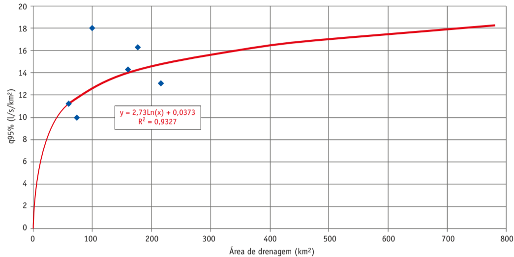
FIGURA 3.4.9 - EQUAÇÃO DE REGRESSÃO ENTRE VAZÃO DE 95% DE PERMANÊNCIA E ÁREA DE DRENAGEM
