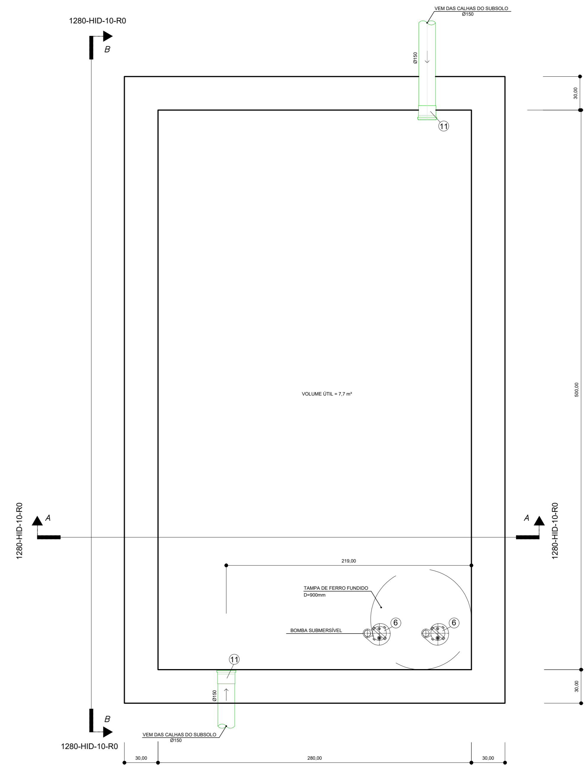
PLANTA BAIXA - RESERVATÓRIO ÁGUAS PLUVIAIS ESCALA 1:20
