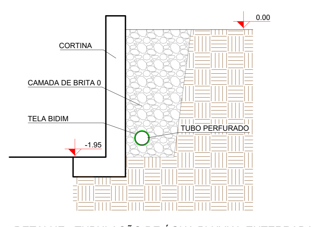
DETALHE - TUBULAÇÃO DE ÁGUA PLUVIAL ENTERRADA ESCALA 1:30
