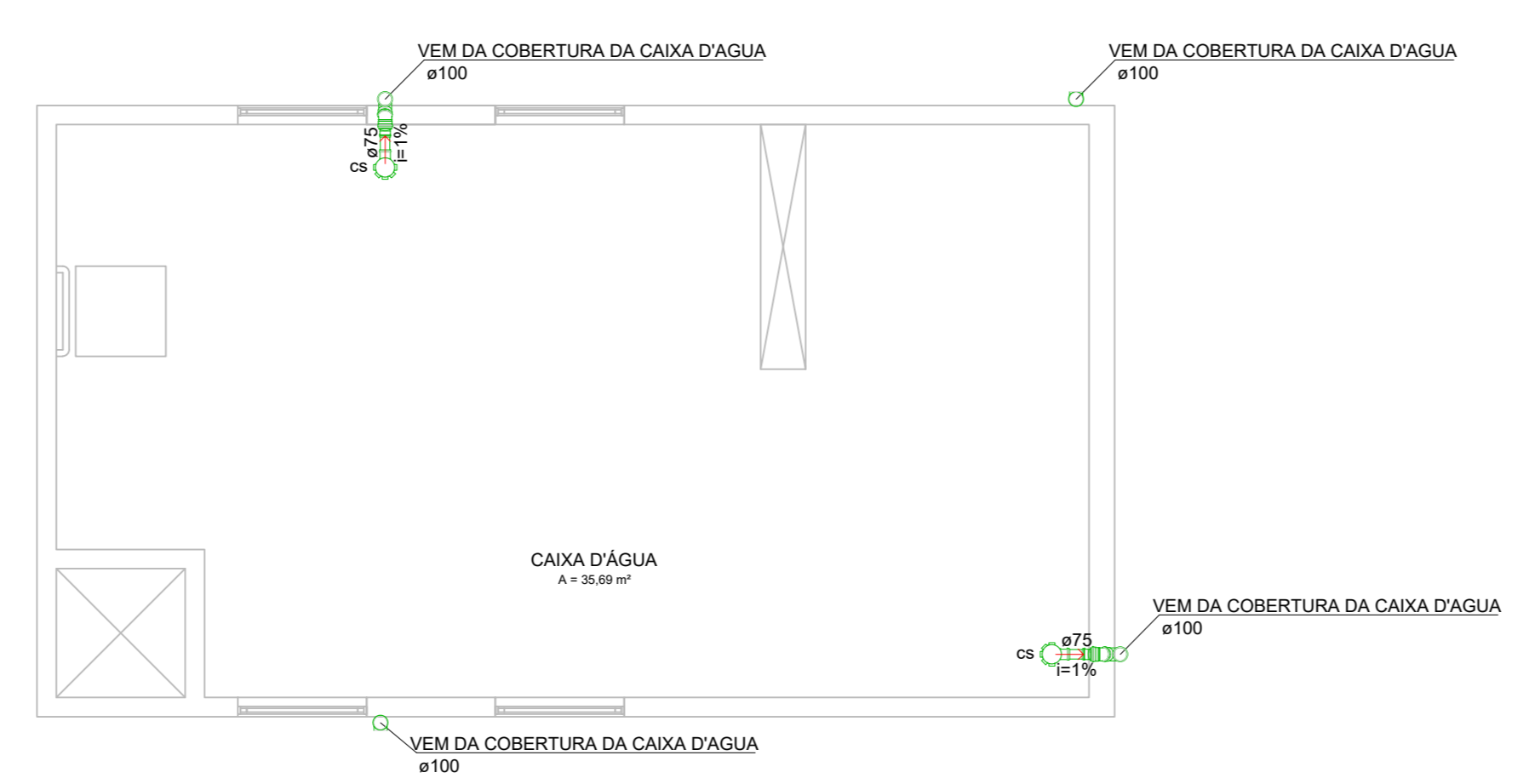
PLANTA BAIXA - CAIXA D'ÁGUA ESCALA 1:50
