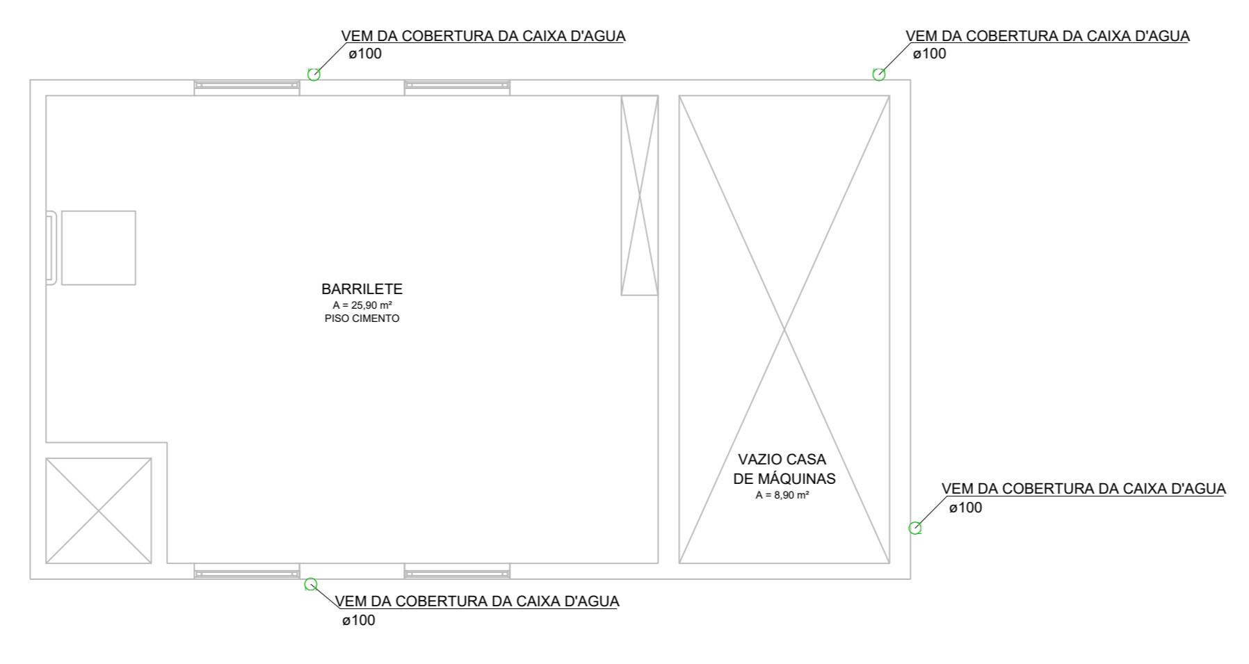
PLANTA BAIXA - BARRILETE ESCALA 1:50
