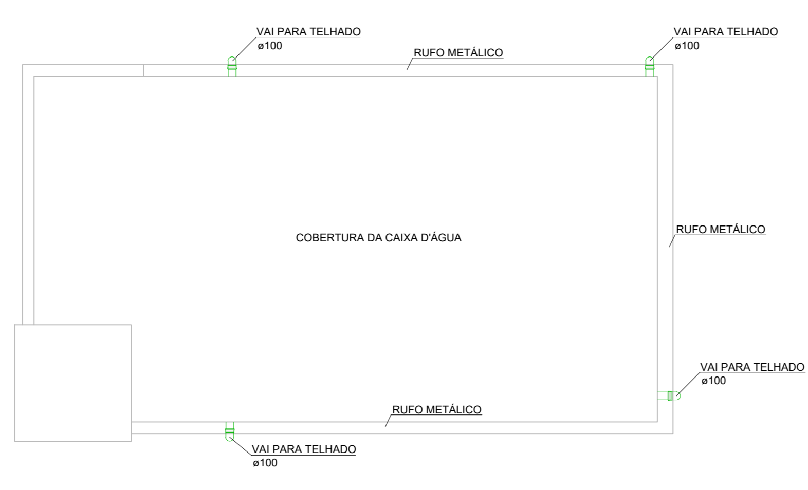
COBERTURA - CAIXA D'ÁGUA ESCALA 1:50
