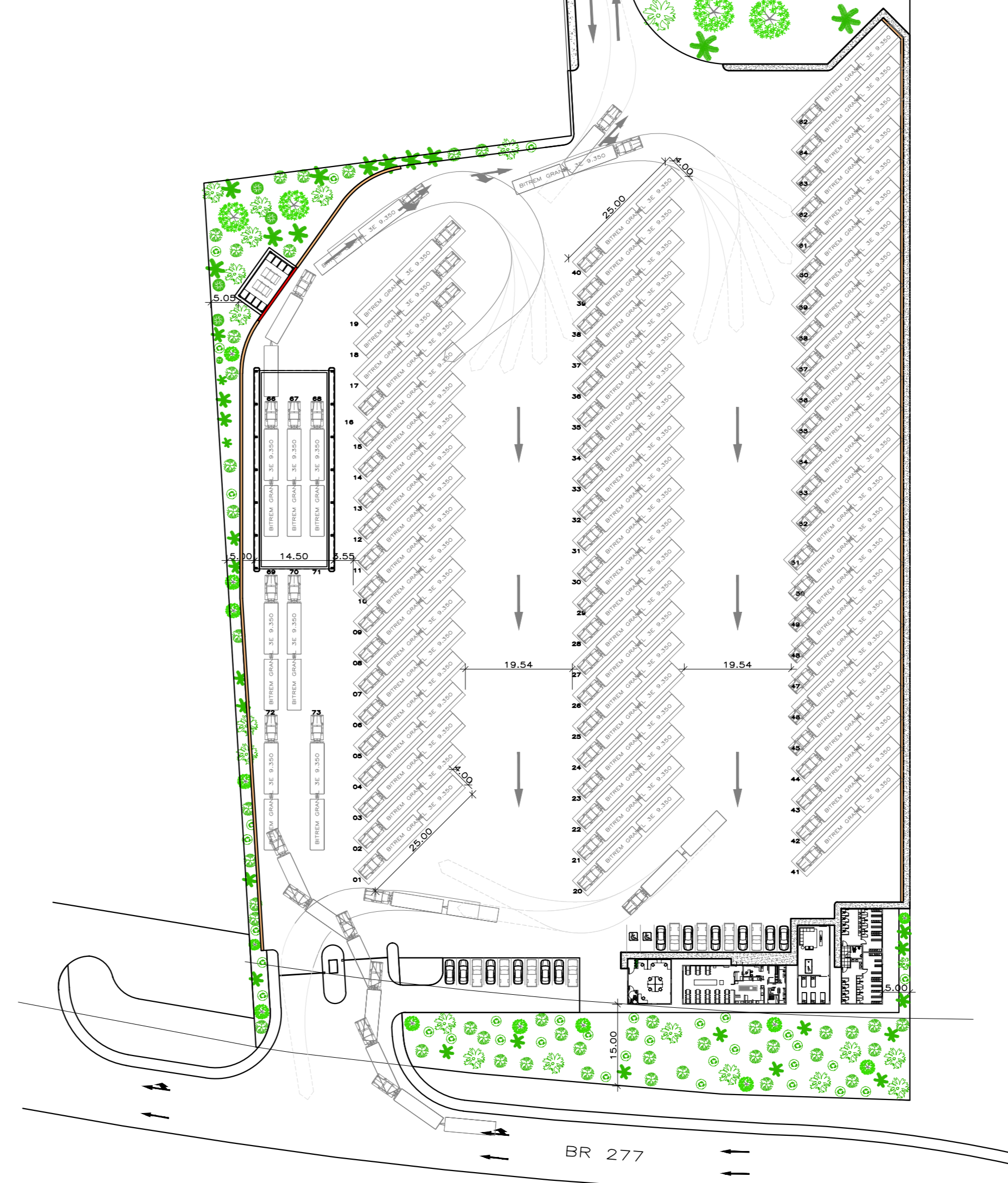
PLANTA DE LOCAÇÃO/LAYOUT DO ESTACIONAMENTO ESCALA: 1:750
