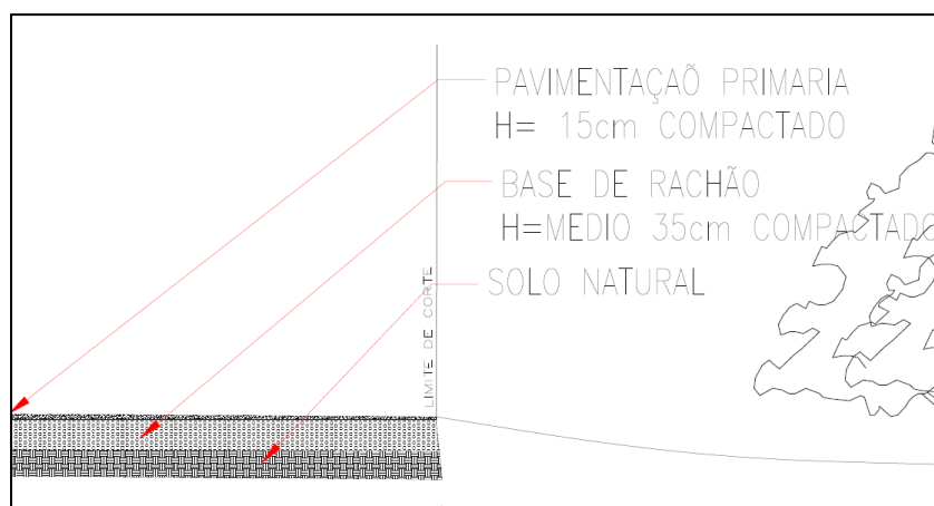
Figura 18: Detalhe da pavimentação prevista no projeto arquitetônico. Fonte: Projeto arquitetônico.
