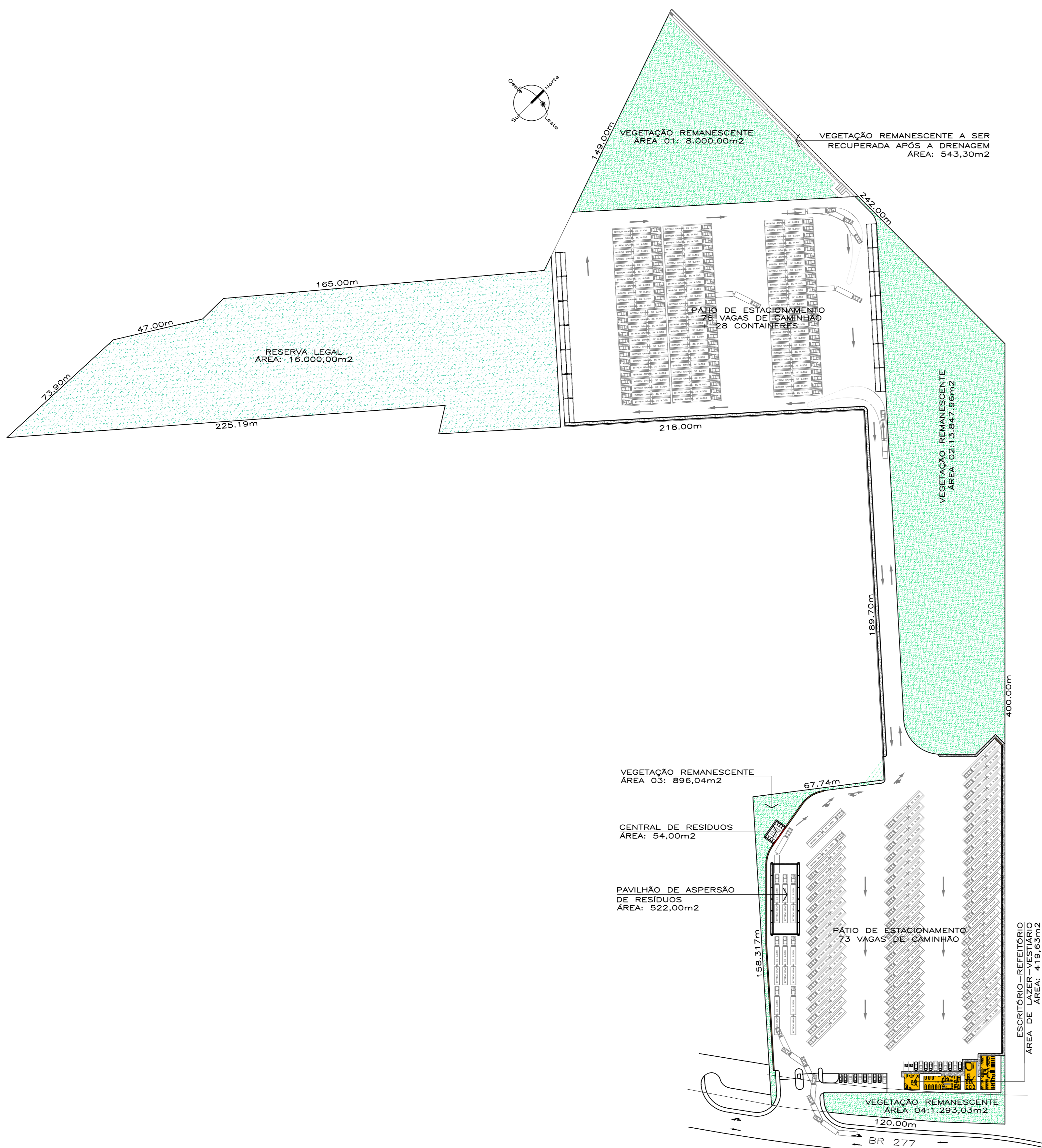
IMPLANTAÇÃO ESC.: 1:1250
