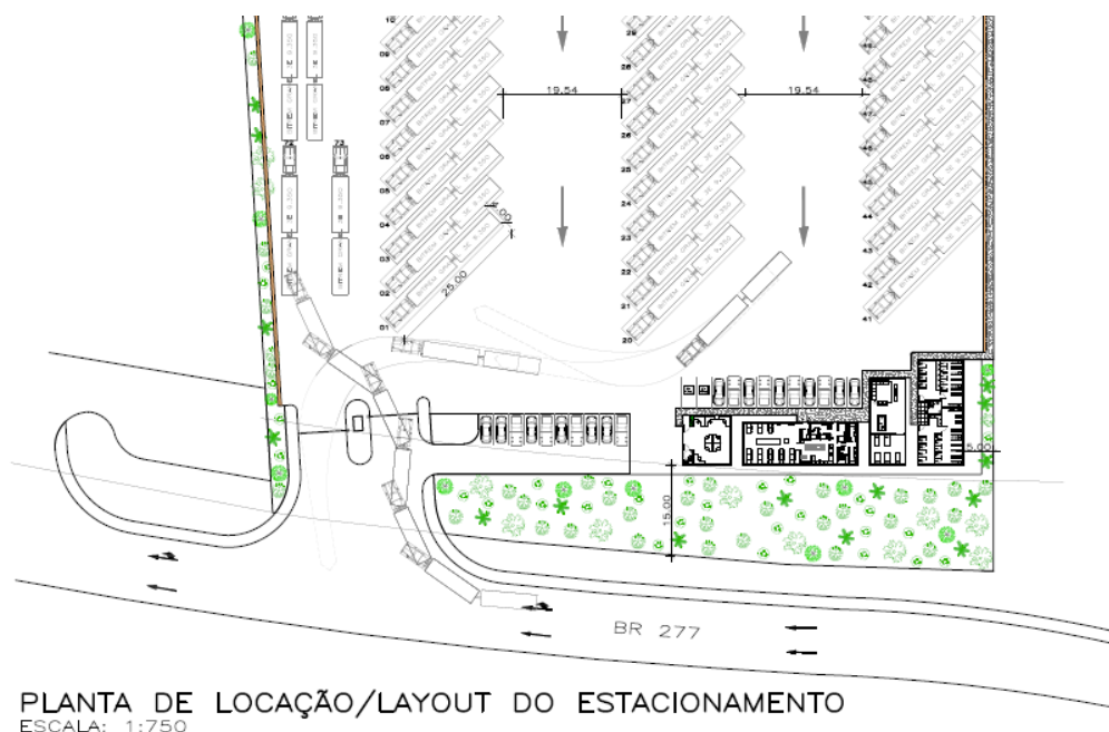
Figura 20: Detalhe do projeto em que se observa o acesso e a saída do empreendimento proposto. Fonte: Planta de Locação.
