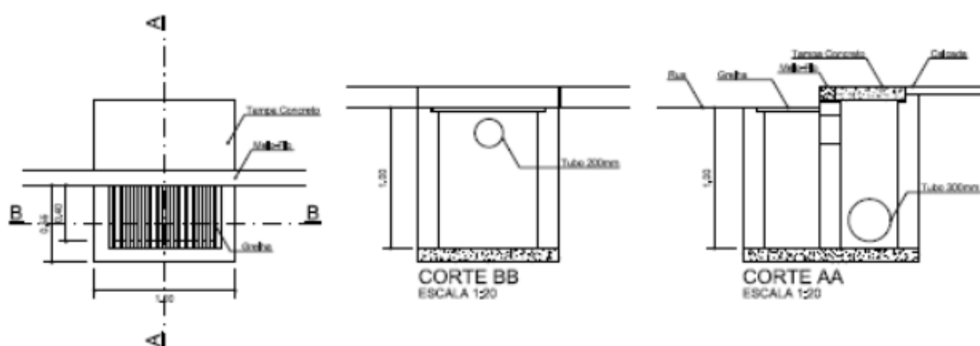
Figura 83: Bueiro ecológico
